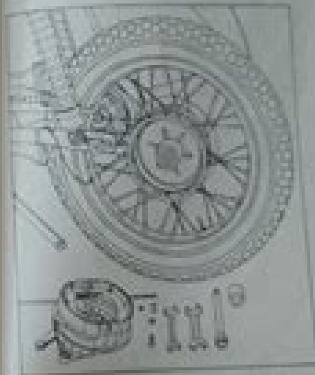
Desmontaje de la rueda trasera, 2.ª fase
