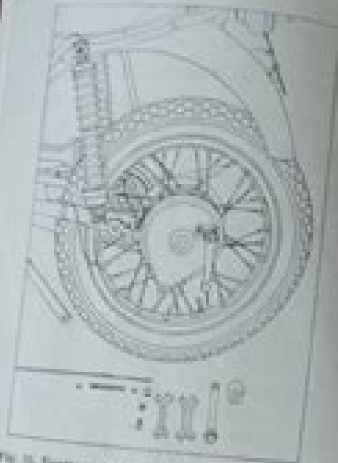
Fig. 24. Desmontaje de la rueda trasera, 1.ª fase
