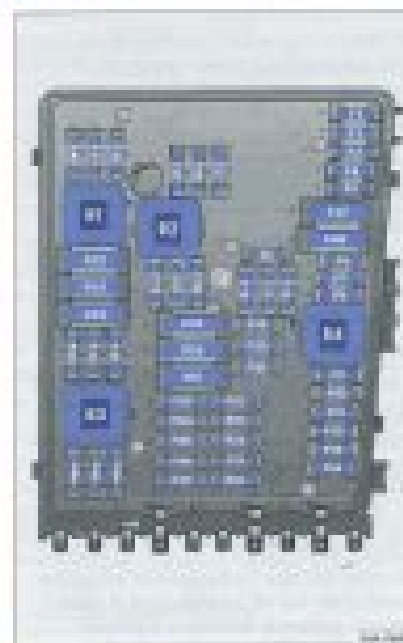
Fig. 42 Fusibles de la caja de fusibles del vano motor Versión B (High End)
