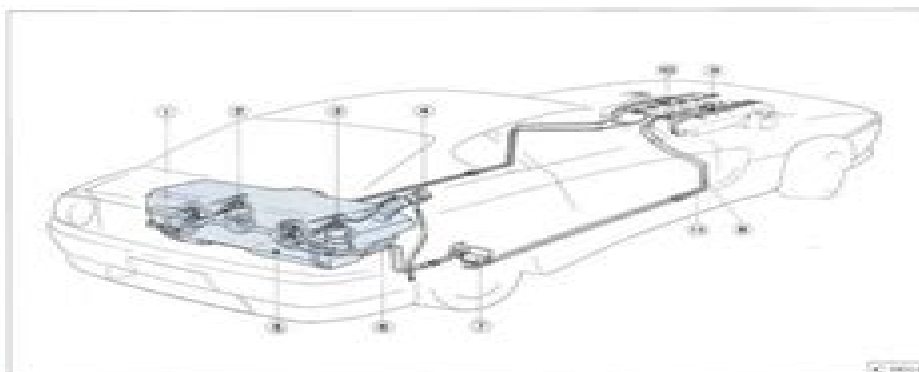
Electrovalvole controllo emissioni vapori benzina
