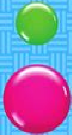
Atoms
