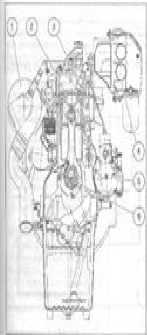
O 2000 MXP (1) Турбонагнетатель (2) Коллекторный канал впускной (3) Клапан дроссельный впускной (4) Система впрыска топлива (5) Вентилятор охлаждения (6) Ремень привода ГРМ
